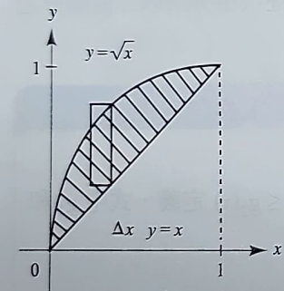
圖 9.12(a) 固定 x 之值， y 的範圍是 x \leq y \leq \sqrt{x} 。
