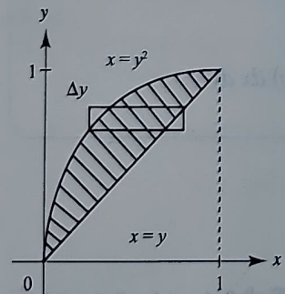
圖 9.12(b) 固定 y 之值， x 的範圍是 y^2 \leq x \leq y 。
