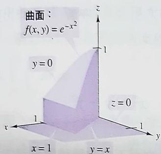
圖 9.17 以 y = 0 ， y = x 和 x = 1 為界的基礎。
