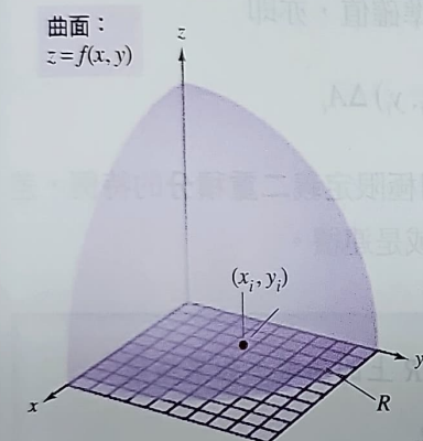
圖 9.7 在 R 內的長方形形成 R 的一個內部分割。
