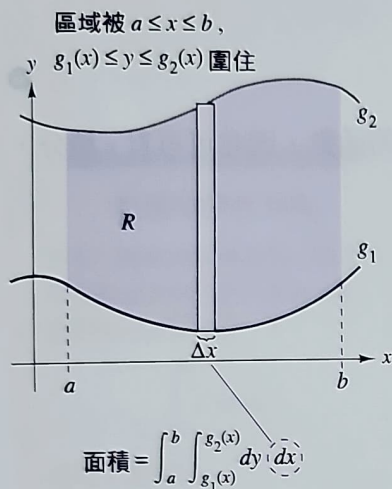
圖 9.2 垂直方向簡單的區域。
