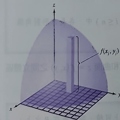
圖 9.8 長方柱體的底面積是 \Delta A_i ，高是 f(x_i, y_i) 。
