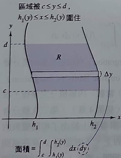
圖 9.3 水平方向簡單的區域。
