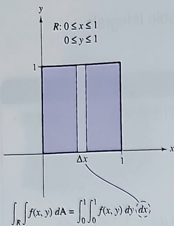
圖 9.11 立體區域的體積是 \frac{2}{3} 。
